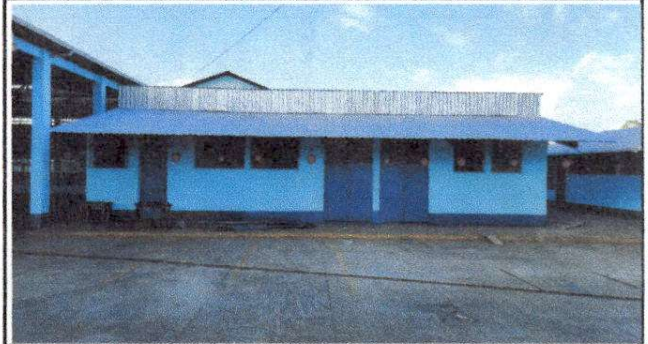
Foto 8: Sustrucción de lámina, por lámina troquelada aluzinc calibre 26 en módulo 4
