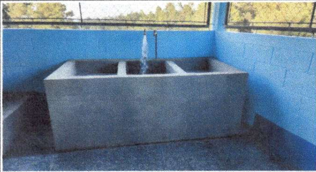
Foto 7: Sustrucción de pila de cemento de dos lavaderos por pila de concreto fundida en módulo 2 cocina
